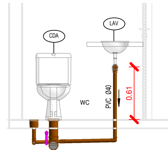
VISTA 02' - ESGOTO 1 : 25
