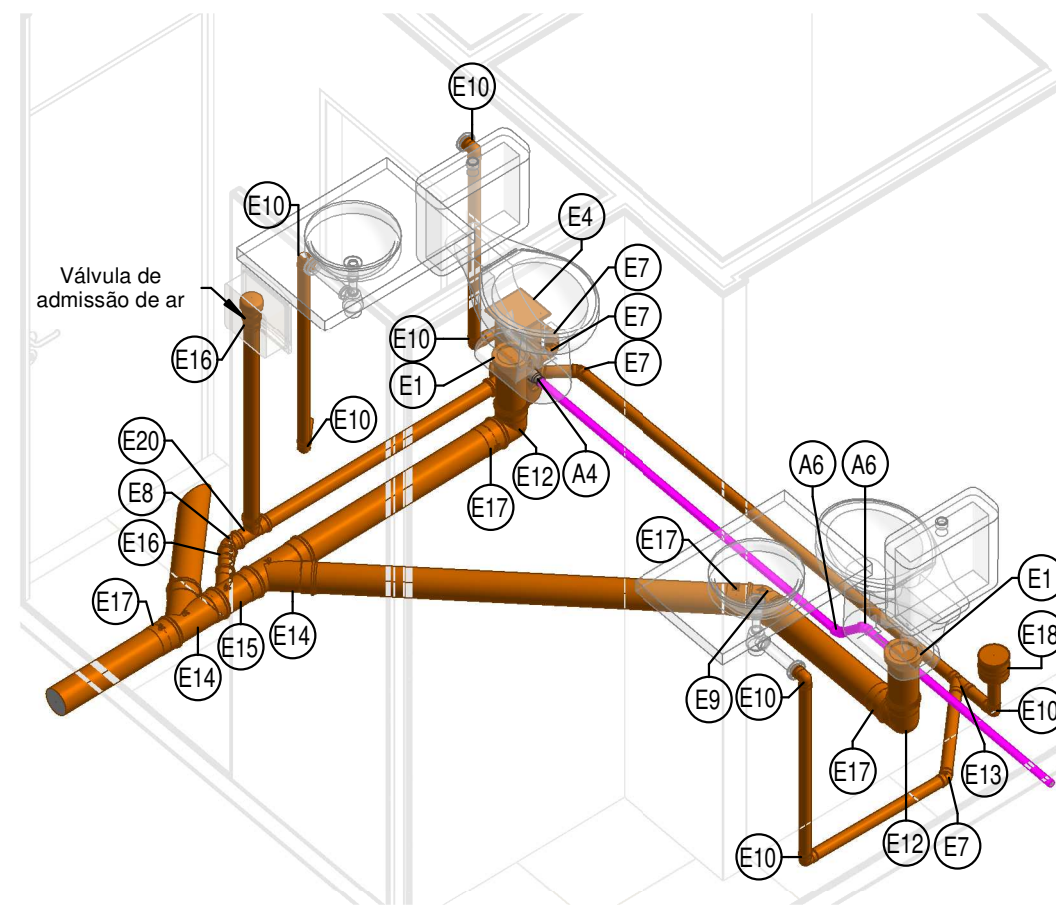
PERSPECTIVA 02 - ESGOTO
